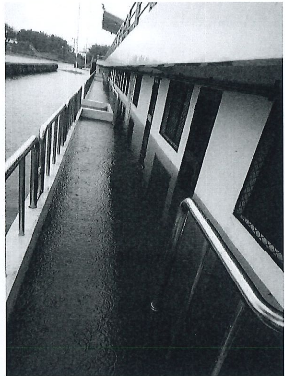
司令台上雨水無法暢通，傾注至司令台下 空間造成積水約 120 公分深
